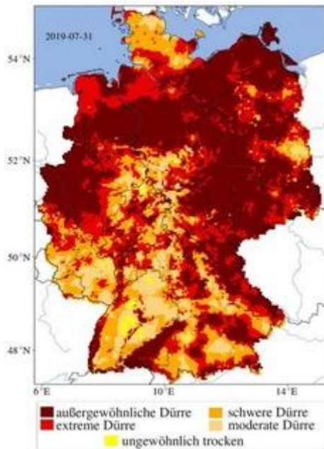
Bild 2. In Fernsachrichten wurden Ende Juli 2019 Bilder wie dieses gezeigt, welche die schlimme Trockenheit unserer Böden selbst noch in einer Tiefe von 1,8 m belegen sollen (Bild: UFZ )
