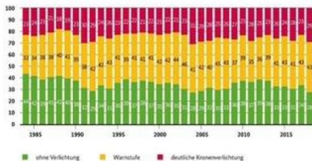
Bild 5. Ergebnisse der Waldzustandserhebung aus den Jahre 1984 bis 2018 (Grafik: BMEL )
